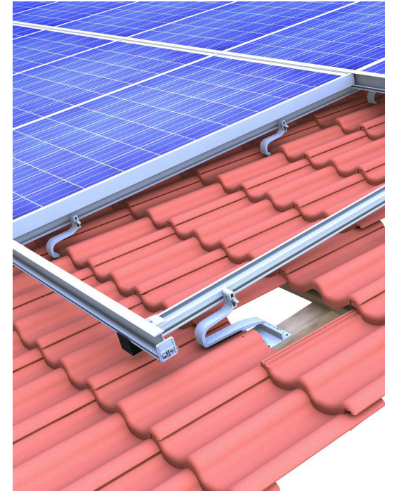
ZD 30 N35 vertical avec rail en C-N comme rail vertical et rail d'insertion
